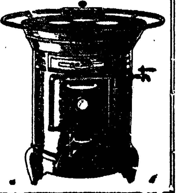
A FORNALHA DAKO PERMITE O APROVEITAMENTO INTEGRAL DO CARVÃO. O QUE NÃO PENETRA PELA CAMARA ADEQUADA, PRODUZINDO A COMBUSTÃO INTEGRAL DOS GAZES
