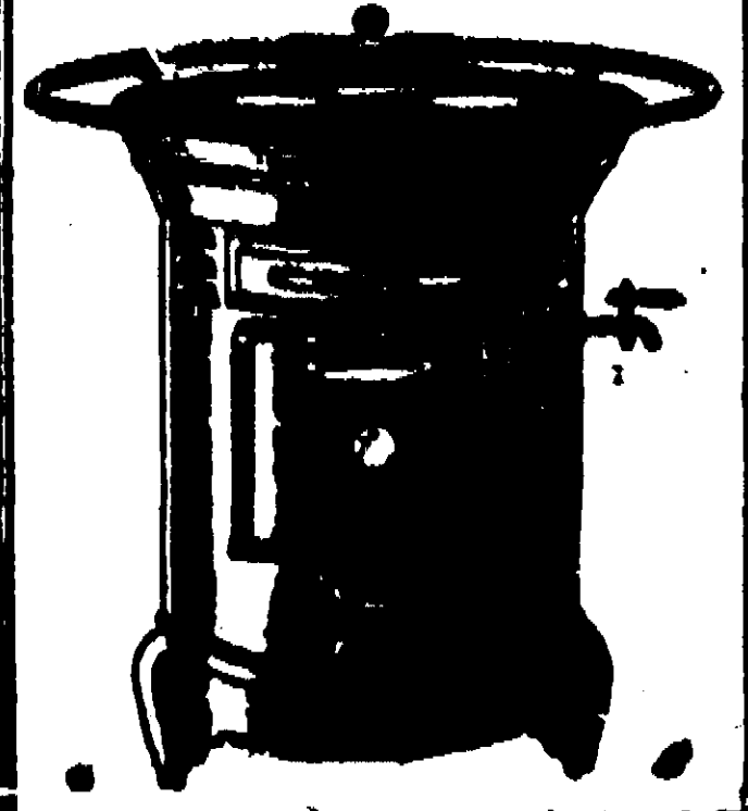
A PORTALHA BARRA PERMITE O APROVEITAMEN-TO INTEGRAL DO CARVÃO. O EXCESSO PENETRA PELA CÁMARA ADEQUADA, PRODUZINDO A COM-BUSTÃO INTEGRAL DOS GAZES.
