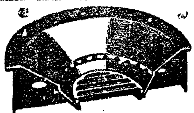
A FORNALHA DAKO PERMITE O APROVEITAMENTO INTEGRAL DO CARVÃO. O OXIGENIO PENETRA PELA SARRANA ADEQUADA, PRODUZINDO A COMBUSTÃO INTEGRAL DOS GAZES
