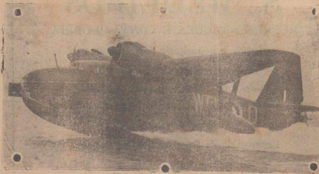
ESTÃO VELANDO PELA SEGURANÇA DOS VAPORES BRITANICOS — Um hydro-avião "Lerwick" bombardeiro e reconhecimento de longo alcance e bem armado, tendo 3 torretes operadas eletricamente com metralhadoras múltiplas
